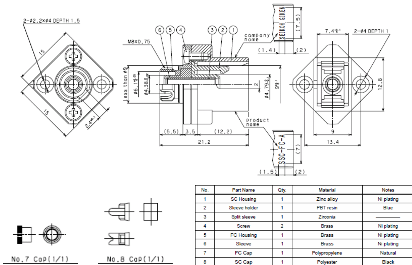
Fig. 1 構造図
