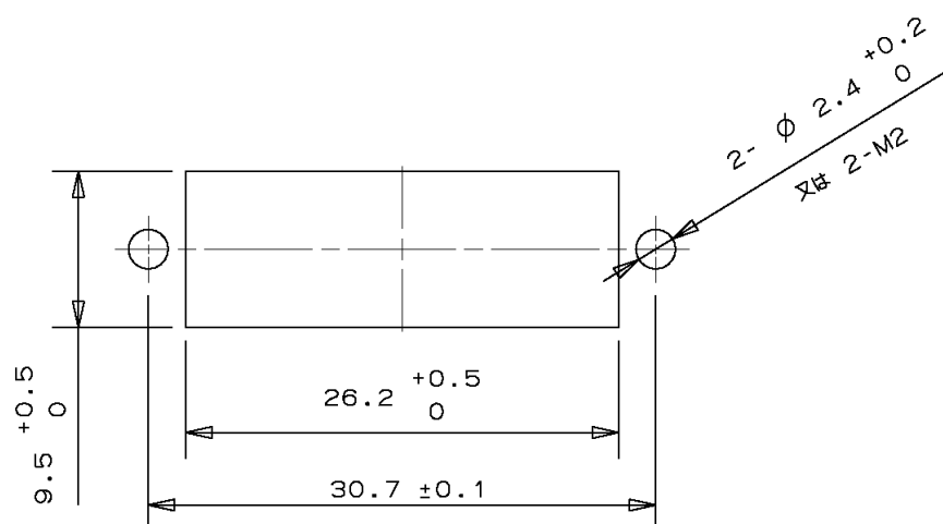
図 4. 取付穴寸法 (参考)
