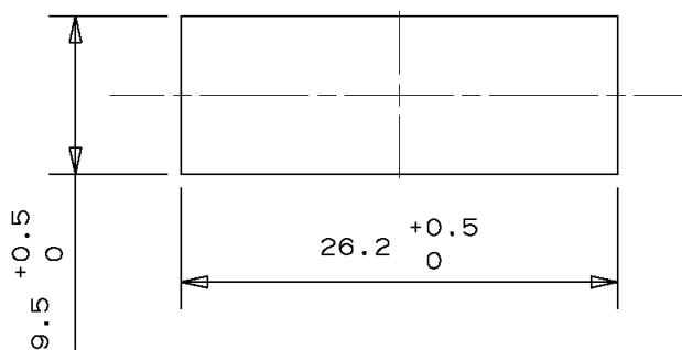
図 4. 取付穴寸法 (参考)
